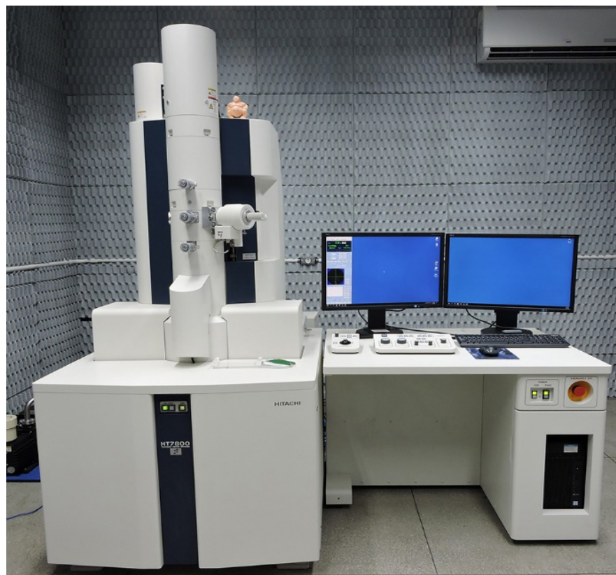
Microscópio Eletrônico de Transmissão Hitachi HT 7800. / Transmission Electron Microscope Hitachi HT 7800.
